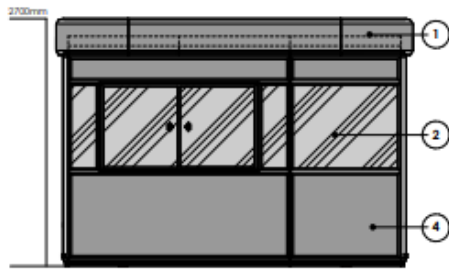
SIDE 2 ELEVATION 1:25
